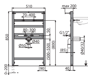
A104/850 Монтажная рама для умывальника
