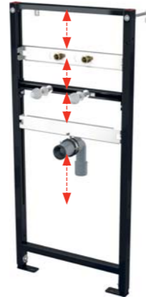
A104A/1120 Монтажная рама для умывальника и смесителя
