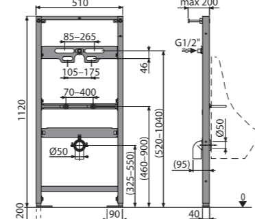
A107/1120 Монтажная рама для писсуара
