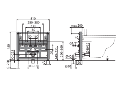
A105/450 Монтажная рама для биде
