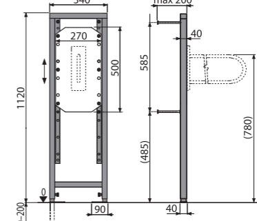
A106/1120 Монтажная рама для поручней
