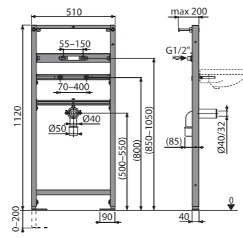
A104A/1120 Монтажная рама для умывальника и смесителя
