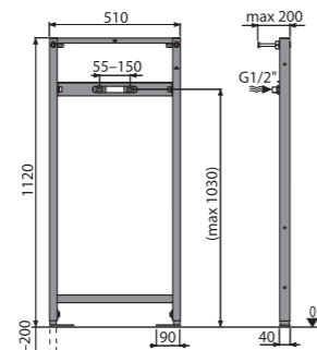
A104B/1120 Монтажная рама для смесителя
