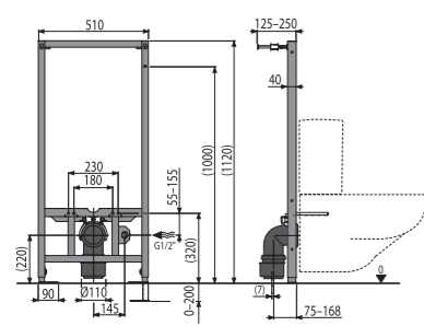
A113/1120 Монтажная рама для подвесного унитаза компакт
