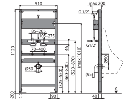
A107S/1120 Монтажная рама для писсуара и сенсорного устройства
