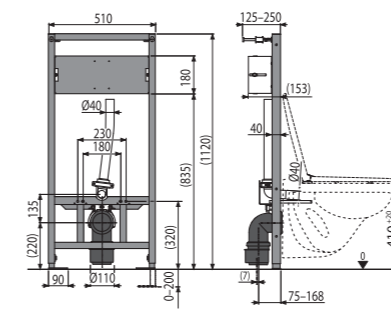
A114S/1120 Монтажная рама для подвесного унитаза и сенсорного устройства
