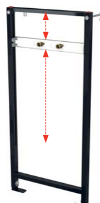
A104B/1120 Монтажная рама для смесителя
