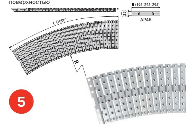
AP4R Решетка для бассейна радиальная с антискользящей поверхностью
